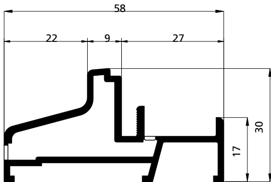
PROFILO PROFIL / PROFIL / PERFIL cod. 3902700
