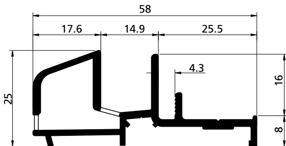
PROFILO PROFIL / PROFIL / PERFIL cod. 3902750
