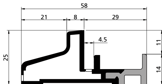
PROFILO PROFIL / PROFIL / PERFIL cod. 3901890
