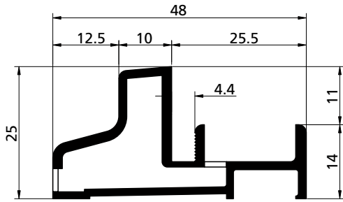
PROFILO PROFIL / PROFIL / PERFIL cod. 3902220
