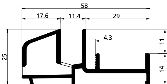
PROFILO PROFIL / PROFIL / PERFIL cod. 3902130
