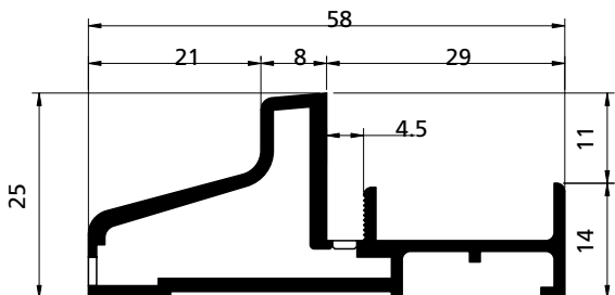
PROFILO PROFIL / PROFIL / PERFIL cod. 3902010
