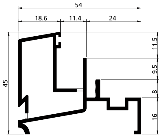
PROFILO PROFIL / PROFIL / PERFIL cod. 3901250
