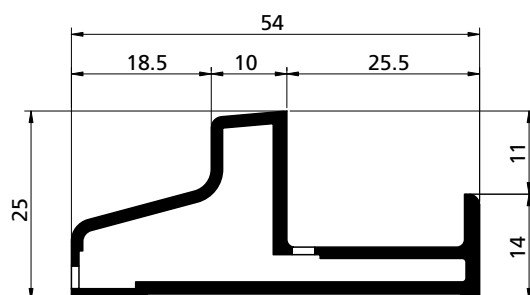
PROFILO PROFIL / PROFIL / PERFIL cod. 3901670
