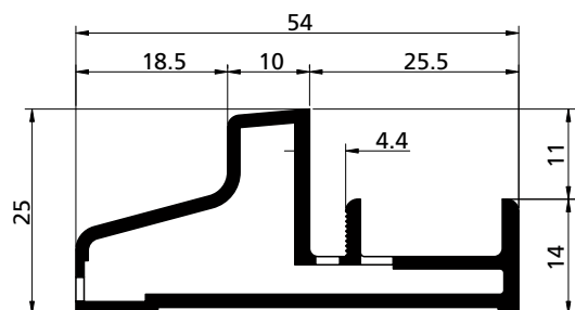
PROFILO PROFIL / PROFIL / PERFIL cod. 3901660
