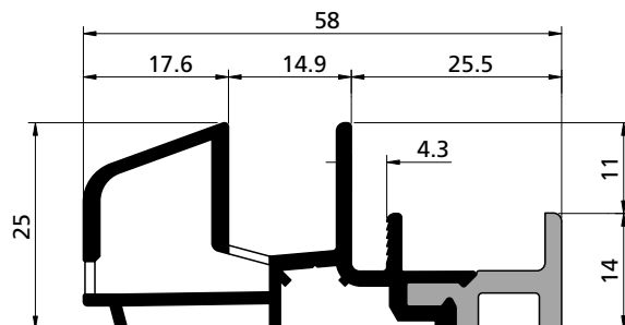
PROFILO PROFIL / PROFIL / PERFIL cod. 3902320
