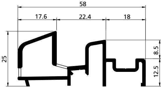
PROFILO PROFIL / PROFIL / PERFIL cod. 3902460
