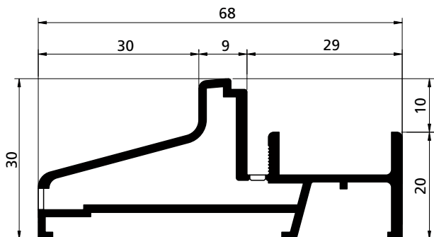
PROFILO PROFIL / PROFIL / PERFIL cod. 3902080
