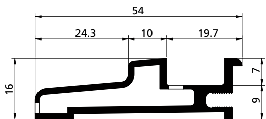
PROFILO PROFIL / PROFIL / PERFIL cod. 3901690
