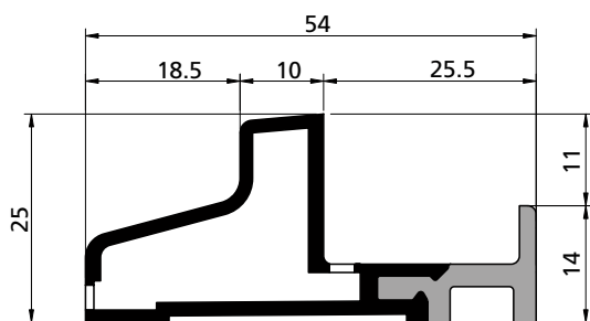
PROFILO PROFIL / PROFIL / PERFIL cod. 3901930
