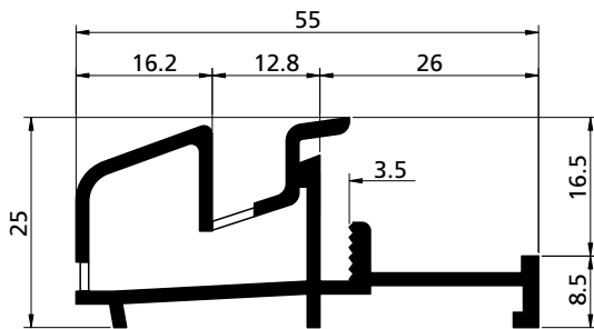
PROFILO PROFIL / PROFIL / PERFIL cod. 41401310
