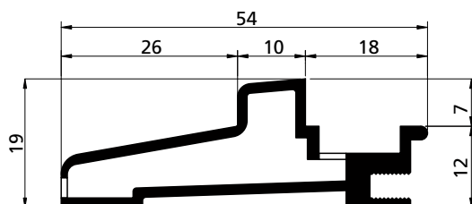
PROFILO PROFIL / PROFIL / PERFIL cod. 3901620
