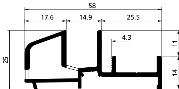
PROFILO PROFIL / PROFIL / PERFIL cod. 3902310
