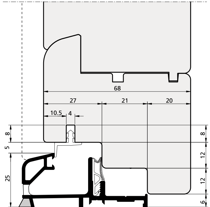
Aria 12 - Battuta 12 Hohraum 12 - Anschlag 12 / Espacement 12 - Butée 12 / Espacio 12 - Antepecho 12
