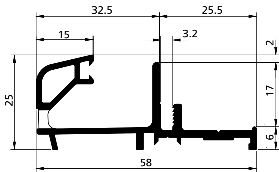
PROFILO PROFIL PROFIL PERFIL cod. 39002890
