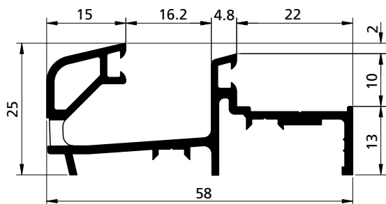
PROFILO PROFIL PROFIL PERFIL cod. 39002990
