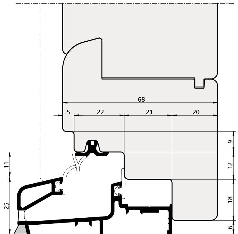
Aria 12 - Battuta 18 Hohraum 12 - Anschlag 18 / Espacement 12 - Butée 18 / Espacio 12 - Antepecho 18
