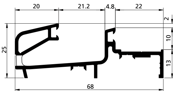
PROFILO PROFIL PROFIL PERFIL cod. 39003010
