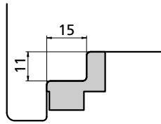
TERMINALE ABSCHLUSS ÉLÉMENT TERMINAL TERMINAL cod. 4001046
