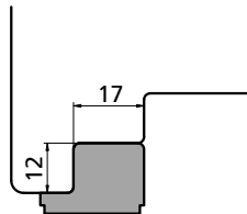
TERMINALE ABSCHLUSS ÉLÉMENT TERMINAL TERMINAL cod. 4001606
