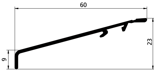
PROFILO PROFIL / PROFIL / PERFIL cod. 3901510
