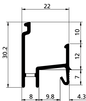
PROFILO PROFIL / PROFIL / PERFIL cod. 3902020
