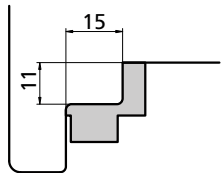
TERMINALE ABSCHLUSS ÉLÉMENT TERMINAL TERMINAL cod. 4001246
