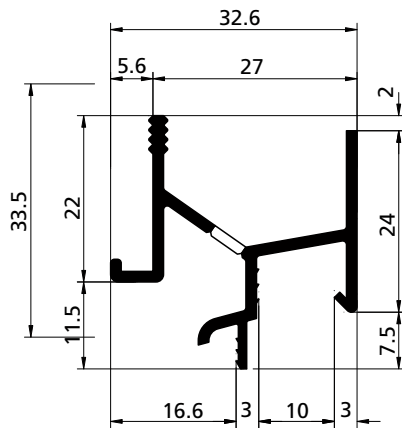
PROFILO PROFIL / PROFIL / PERFIL cod. 3902090
