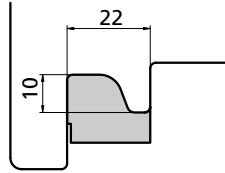
TERMINALE ABSCHLUSS ÉLÉMENT TERMINAL TERMINAL cod. 4001609
