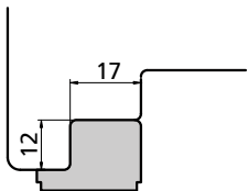
TERMINALE ABSCHLUSS ÉLÉMENT TERMINAL TERMINAL cod. 4001606
