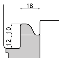
TERMINALE ABSCHLUSS ÉLÉMENT TERMINAL TERMINAL cod. 4001887
