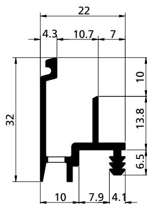
PROFILO PROFIL / PROFIL / PERFIL cod. 3901320
