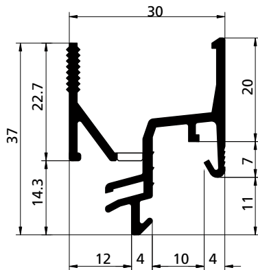
PROFILO PROFIL / PROFIL / PERFIL cod. 3902120
