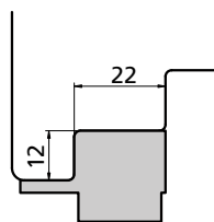
TERMINALE ABSCHLUSS ÉLÉMENT TERMINAL TERMINAL cod. 4002036
