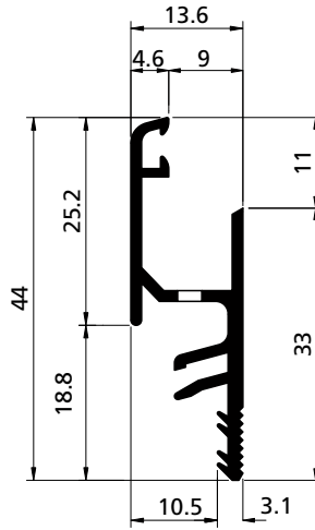
PROFILO PROFIL / PROFIL / PERFIL cod. 3901400
