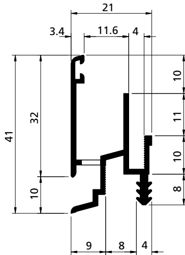
PROFILO PROFIL / PROFIL / PERFIL cod. 3901520
