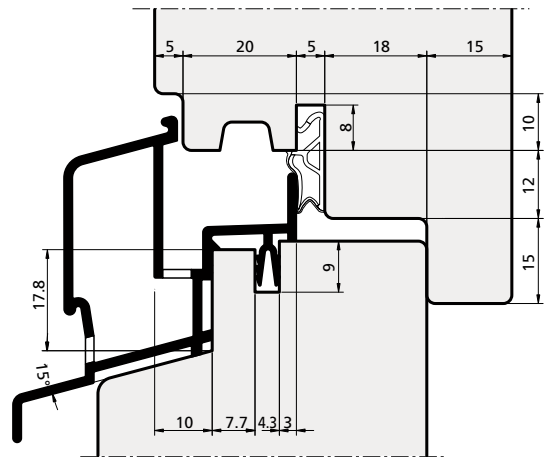
PROFILO PROFIL / PROFIL / PERFIL cod. 39002640
