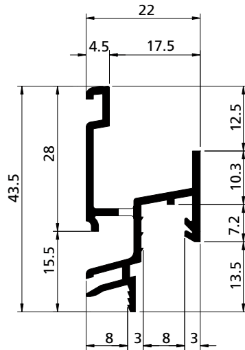
PROFILO PROFIL / PROFIL / PERFIL cod. 3901720
