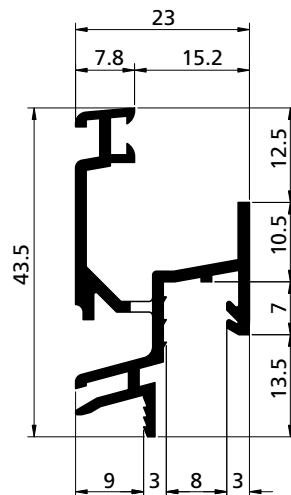
PROFILO PROFIL / PROFIL / PERFIL cod. 3901710
