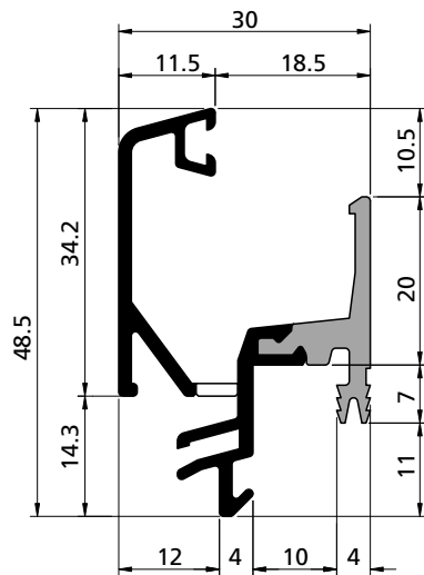
PROFILO PROFIL / PROFIL / PERFIL cod. 3901880
