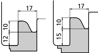
TERMINALE ABSCHLUSS ÉLÉMENT TERMINAL TERMINAL cod. 4001618
