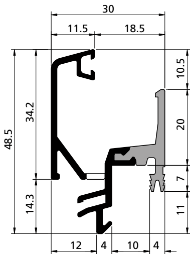
PROFILO PROFIL / PROFIL / PERFIL cod. 3901880
