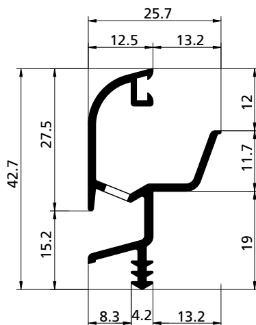
PROFILO PROFIL / PROFIL / PERFIL cod. 3902300
