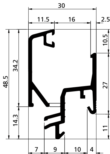
PROFILO PROFIL / PROFIL / PERFIL cod. 3901900
