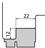
TERMINALE ABSCHLUSS ÉLÉMENT TERMINAL TERMINAL cod. 4002046
