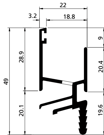
PROFILO PROFIL / PROFIL / PERFIL cod. 3901760
