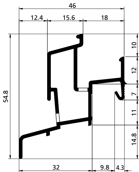
PROFILO PROFIL / PROFIL / PERFIL cod. 3902040
