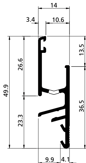
PROFILO PROFIL / PROFIL / PERFIL cod. 3901970
