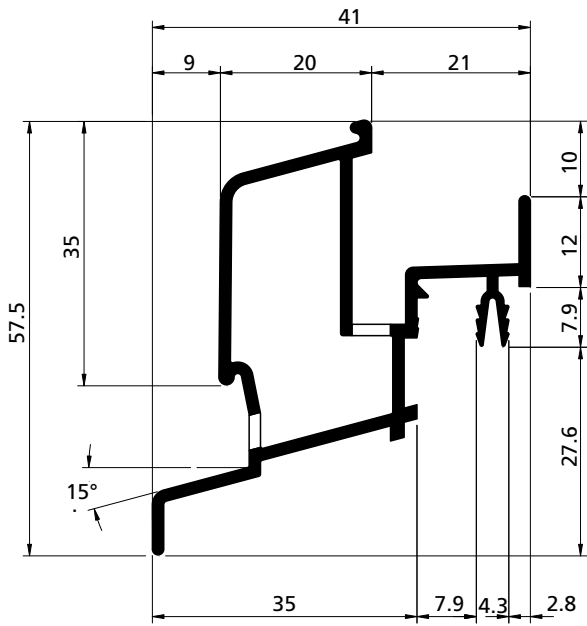
PROFILO PROFIL / PROFIL / PERFIL cod. 39002640
