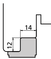
TERMINALE ABSCHLUSS ÉLÉMENT TERMINAL TERMINAL cod. 4001267
