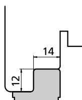
TERMINALE ABSCHLUSS ÉLÉMENT TERMINAL TERMINAL cod. 4001267
