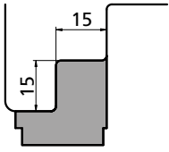
TERMINALE ABSCHLUSS ÉLÉMENT TERMINAL TERMINAL cod. 4002066
