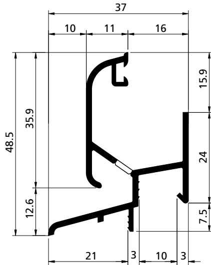
PROFILO PROFIL / PROFIL / PERFIL cod. 3902060
