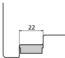
TERMINALE ABSCHLUSS ÉLÉMENT TERMINAL TERMINAL cod. 4002026
