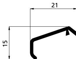
PROFILO PROFIL / PROFIL / PERFIL cod. 3901560
