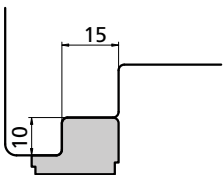
TERMINALE ABSCHLUSS ÉLÉMENT TERMINAL TERMINAL cod. 4001766
