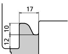
TERMINALE ABSCHLUSS ÉLÉMENT TERMINAL TERMINAL cod. 4001618
