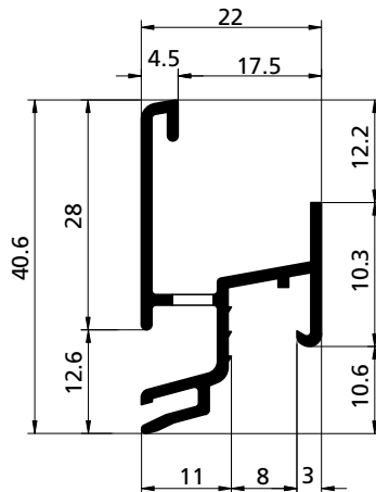
PROFILO PROFIL / PROFIL / PERFIL cod. 3902270
