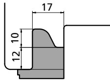
TERMINALE ABSCHLUSS ÉLÉMENT TERMINAL TERMINAL cod. 4002237
