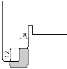
TERMINALE ABSCHLUSS ÉLÉMENT TERMINAL TERMINAL cod. 4001406
