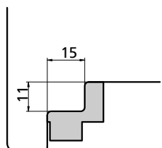
TERMINALE ABSCHLUSS ÉLÉMENT TERMINAL TERMINAL cod. 4001046
