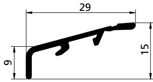
PROFILO PROFIL / PROFIL / PERFIL cod. 3901500
