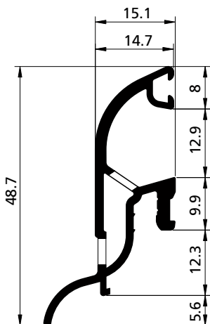
PROFILO PROFIL PROFIL PERFIL cod. 39003190
