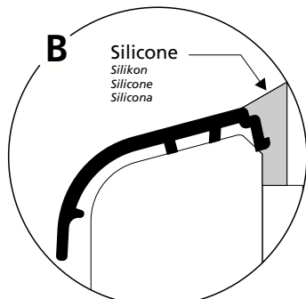
B Variante applicazione profilo cod. 39003200 senza aggancio
