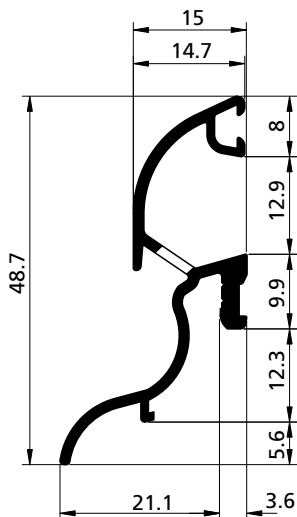
PROFILO PROFIL PROFIL PERFIL cod. 39003070
