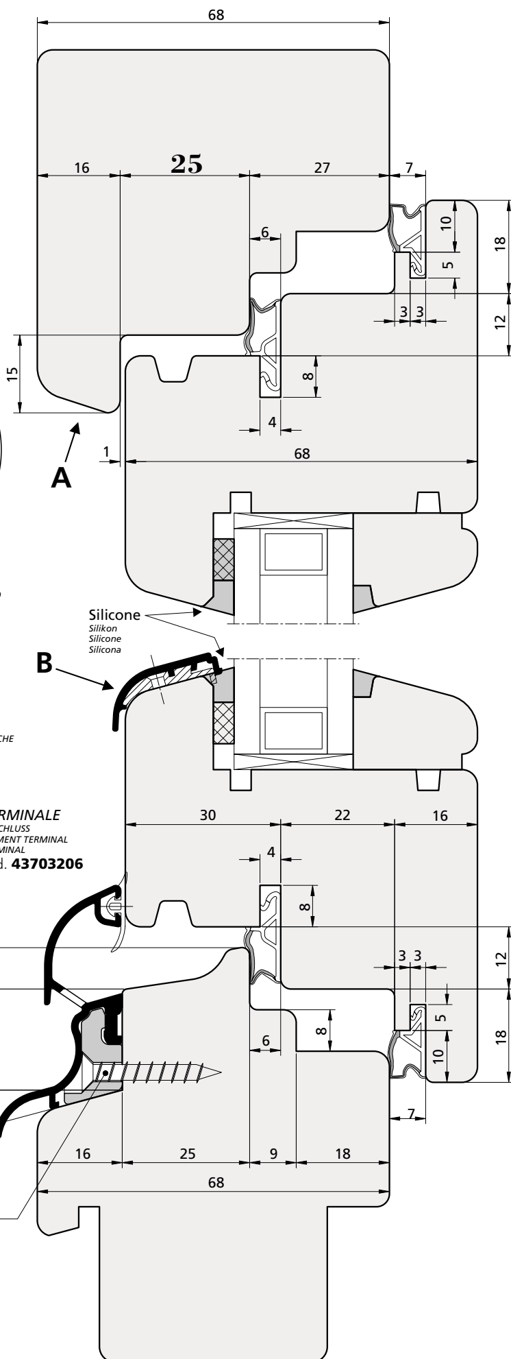
B Variante applicazione profilo cod. 39003200 senza aggancio
