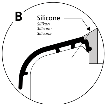
B Silicone Silikon Silicone Silicona Variante applicazione profilo cod. 39003200 senza aggancio Variante Profilanbringung Cod. 39003200 ohne Haken Option d'application de profil cod. 39003200 sans accrochage Variante aplicación perfil cód. 39003200 sin enganche
