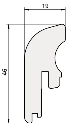
FASCETTA IN LEGNO HOLZSTREIFEN LISSE EN BOIS ABRAZADERA DE MADERA
